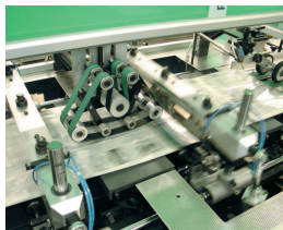
Feeder with singulating disk Mettifooglio con disco separatore
